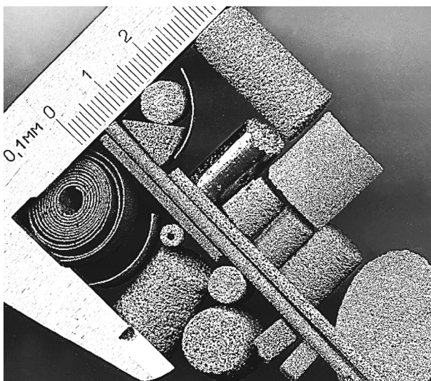
Рисунок 4. Представители четвёртого класса имплантатов из никелида титана – носители клеточных культур [11]
