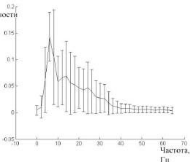
Рисунок 2. Удельное значение спектральной плотности мощности для единичной записи излучения мобильного телефона
