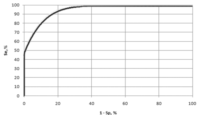
Рис.5. ROC-кривая оценки эффективности прогнозно-диагностической модели
