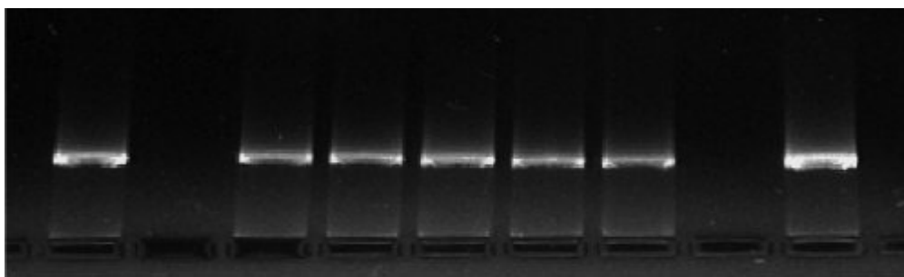
Рис. 4. Электрофореграмма полученная после прямого воздействия на ДНК фага ? исследуемых веществ, смешанных в различных соотношениях. Воздействие при 300С в течение 3 часов и 20 часов при комнатной температуре.
