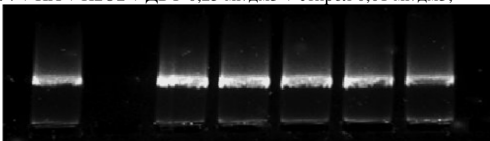
Рис. 5. Электрофореграмма полученная после инкубации в системе метаболической активации ДНК фага ? и исследуемых веществ, смешанных в различных соотношениях.
