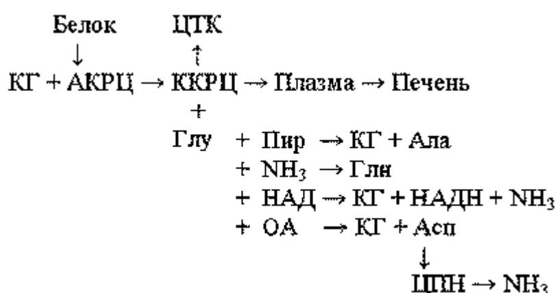
Рис.2. Пути возможного превращения АКРЦ и их аминокислот. Сокращения: КГ (кетоглутарат), Глу (глутамин), Пир (пируват), Ала (аланин), Глн (глутамин), ОА (оксалоацетат), Асп (аспартат)
