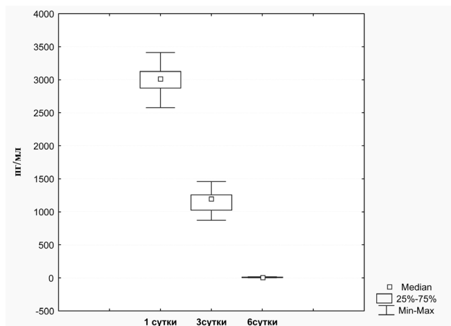
Рисунок 2 -Концентрация тромбоцитарного фактора роста-BB в культуре фибробластов кожи человека в среде с 10% обогащенной тромбоцитами плазмой на 1, 3 и 6 сутки культивирования
