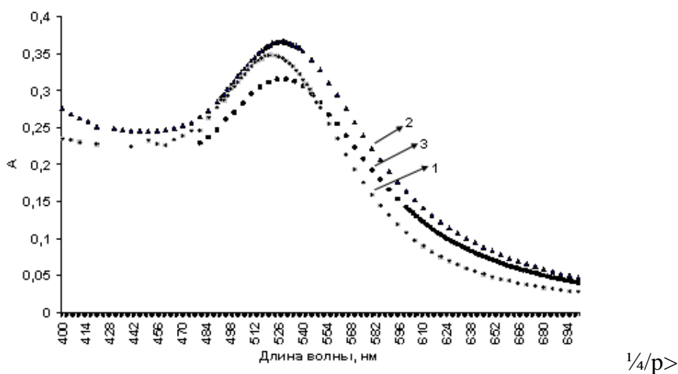
Рисунок 1 – Спектры поглощения исходного золя золота (1), золя, стабилизированного антителами (2) и после добавления NaCl (3)
