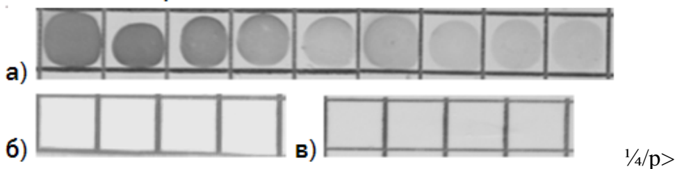
Рисунок 2 – иммунозолотой дот-анализ дифтерийного анатоксина (а), БСА (б), среды пгла MEM (в).
