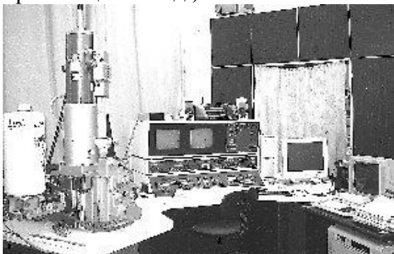
Рис.2. Сканирующий электронный микроскоп CamScan 4 с микрорентгеноспектральным анализатором AN 10000
