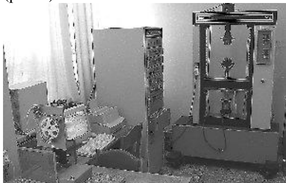
Рис.1. Комплекс механических испытаний на базе испытательной машины Instron-1195 и копра КМ-04
